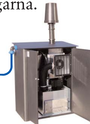
CTS 2000-E förbränningsanläggning som bränner med elektricitet.
